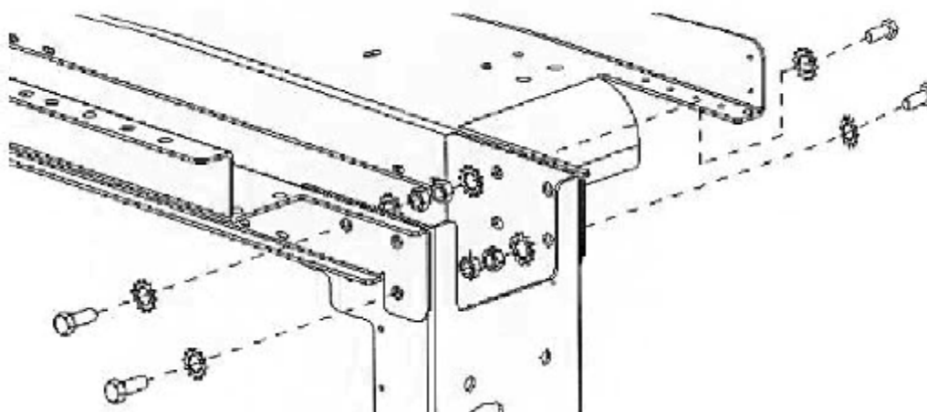
图19 典型的机柜组合硬件
