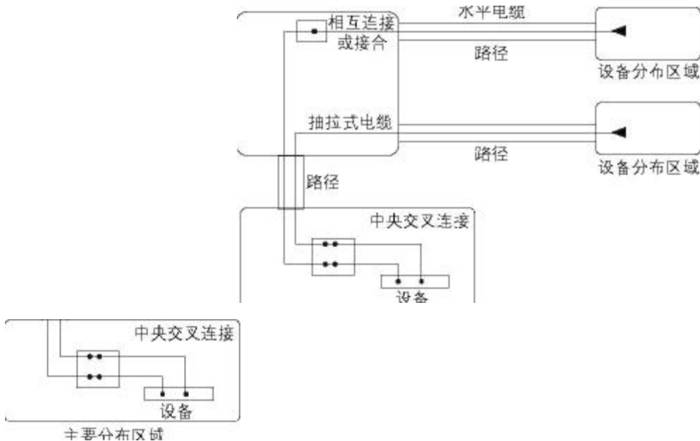
图9 中心光纤电缆
