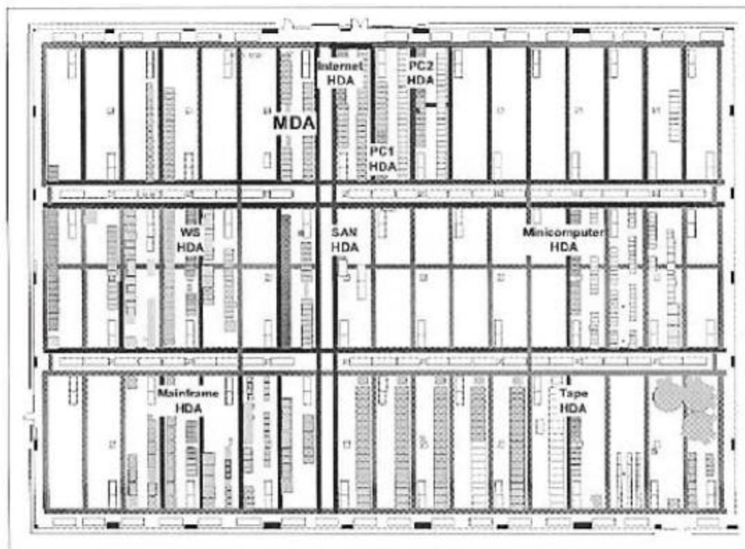
(图 21：公司数据中心范例)
