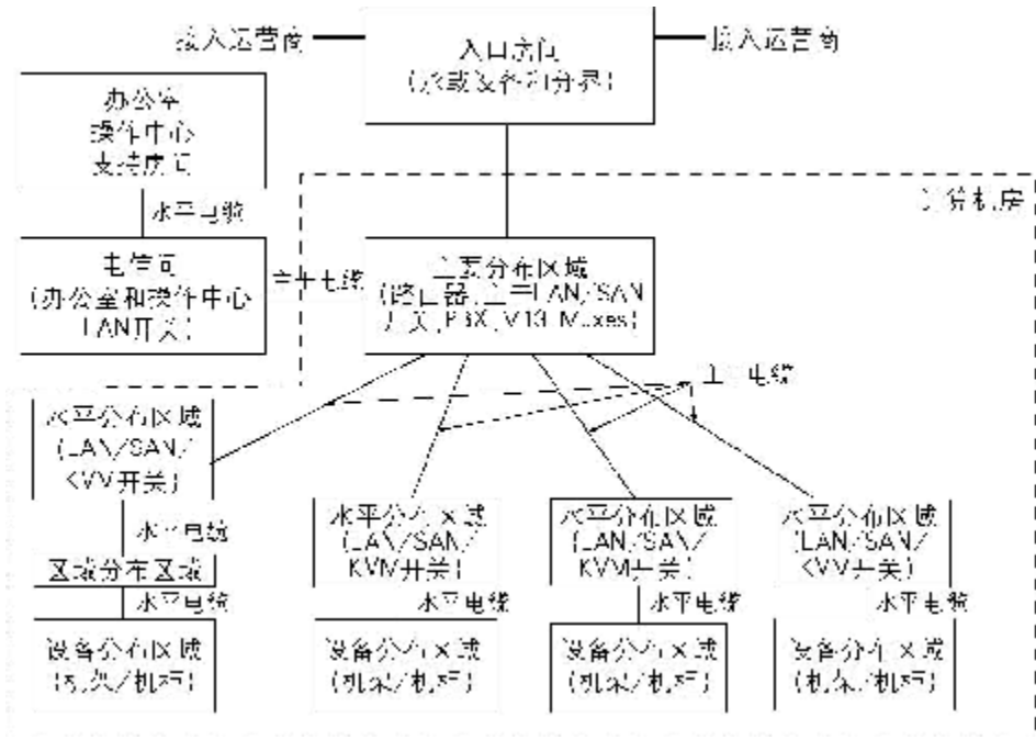
图3 基本的数据中心布局范例的机柜或机架那么小。在一个简化的数据中心布局中，用于电缆连接支持区域和入口房间的电信机房也可以被合并到主要分布区域中。图4所表示是针对小型数据中心的简化数据中心布局。接入运营商
