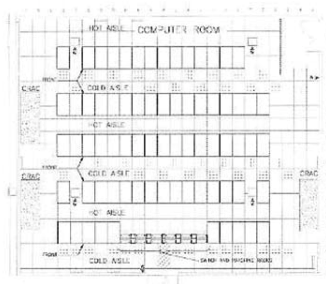
（图20：显示“热”和“冷”通道的计算机房规划图）
