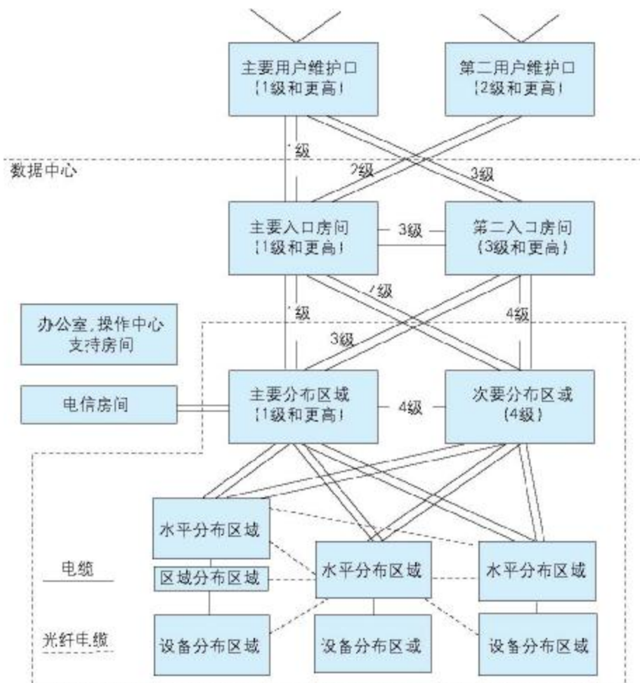
图10 电信基础设施冗余
