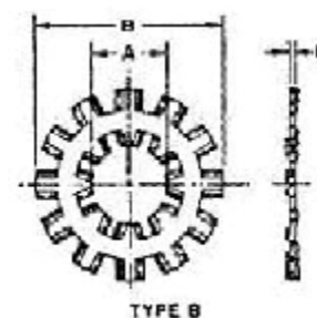
图18美国标准的内部至外部的 齿锁垫圈(ASA B27.1-1965), 类型B
