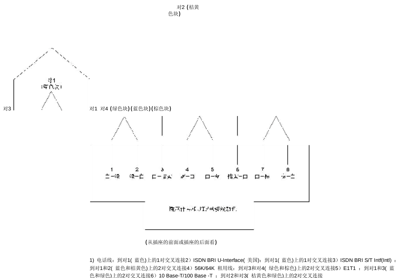
图16 IDC连接硬件电缆到模块插座在T568A 8针顺序的交叉连接电路
